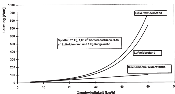
Abbildung 1: Abhängigkeit der zu überwindenden Widerstände beim Radfahren mit zunehmender Geschwindigkeit. Der größte Bremswiderstand geht vom Luftwiderstand aus. Rollwiderstand und Hangabtriebskomponente sind auf der Ebene von untergeordneter Bedeutung (modif. nach 6).
